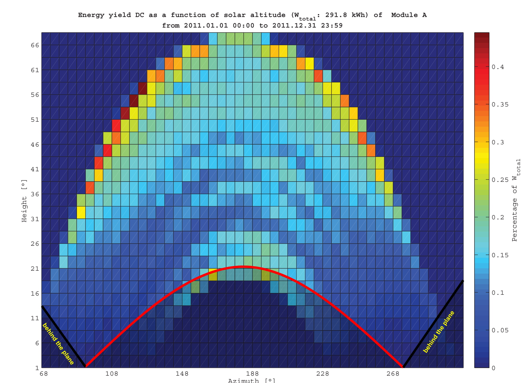
Abbildung 3: Jährlicher Energieertrag des Referenzmoduls ( P_{DCflash} = 226.2 \text{ W} ) für unterschiedliche Positionen des Sonnenstandes in Abhängigkeit von Azimut und Sonnenhöhe für das Messjahr 2011 (Neigung 30°, Süd). Die rote Linie zeigt die Abschattung bei Abschattungswinkel 20°.
