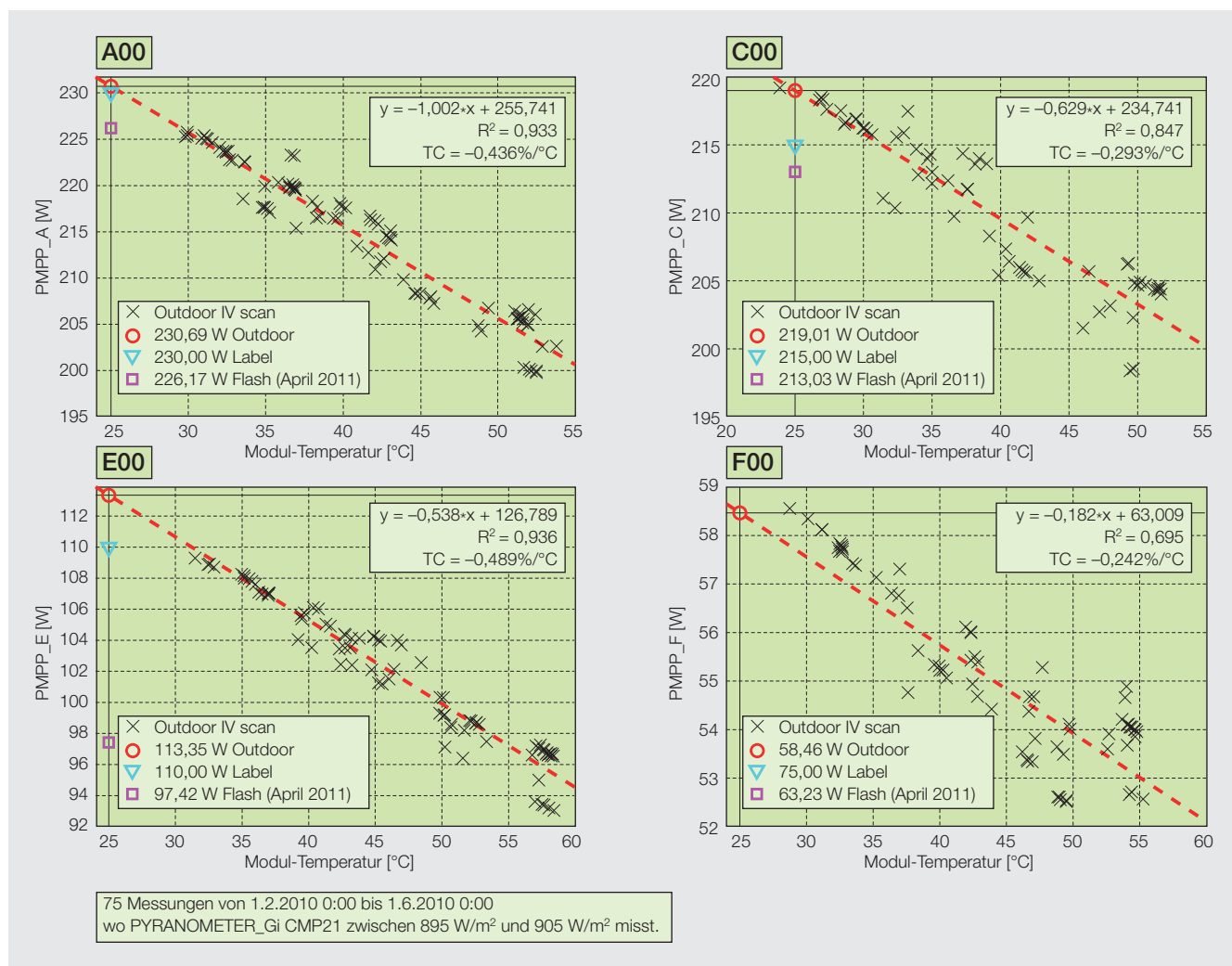
Bild 3 Bestimmung des Temperaturkoeffizienten (TC) der Nennleistung (Tabelle 1) und der STC-Modulnennleistung durch Sortierung der Outdoor-Messdaten im Einstrahlungsintervall von 895 bis 905 W/m² (Leistungsschse linear auf STC skaliert).
