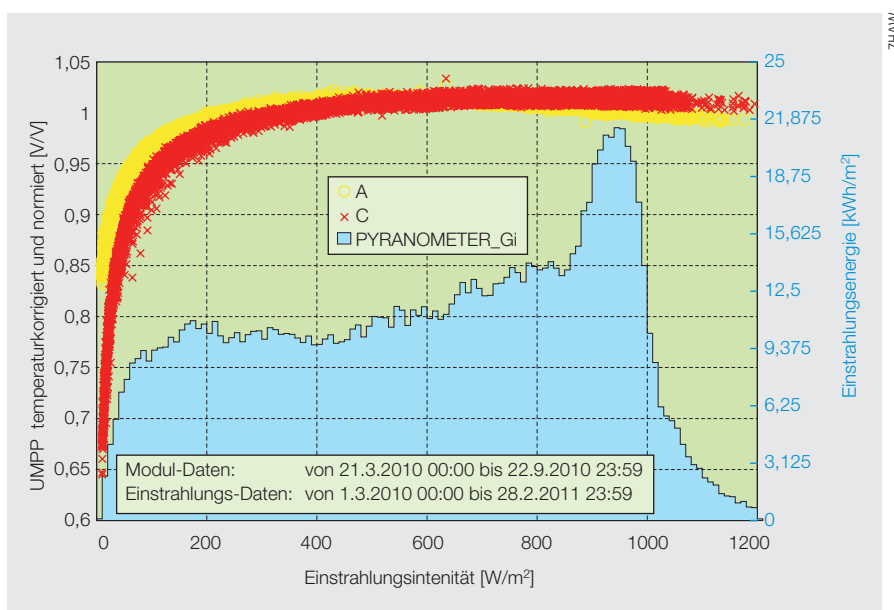
Bild 5 Schwachlichtverhalten der Spannung im MPP auf 25 °C bezogen und die Flashermessung im April 2011 am Beispiel von Typ A und Typ C. Dabei wurde der Temperaturkoeffizient linear mit der Einstrahlungsleistung berechnet. Zusätzlich wurde die Häufigkeitsverteilung der gemessenen Jahreseinstrahlungssumme in der geeigneten Ebene dargestellt.
